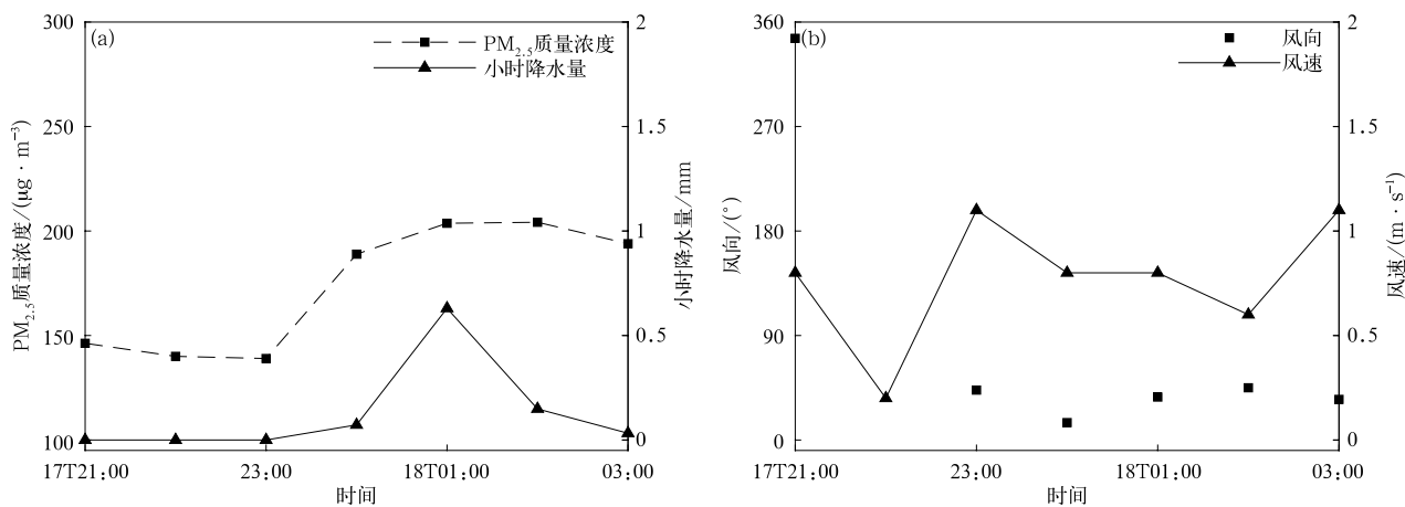
图11 2015年9月17—18日北京小雨过程 \text{PM}_{2.5} 质量浓度和小时降水量(a)以及风速和风向(b)随时间变化
