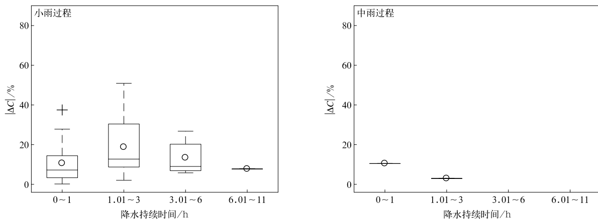
图7 2014年3月—2016年7月北京降水后 PM_{2.5} 质量浓度增加
