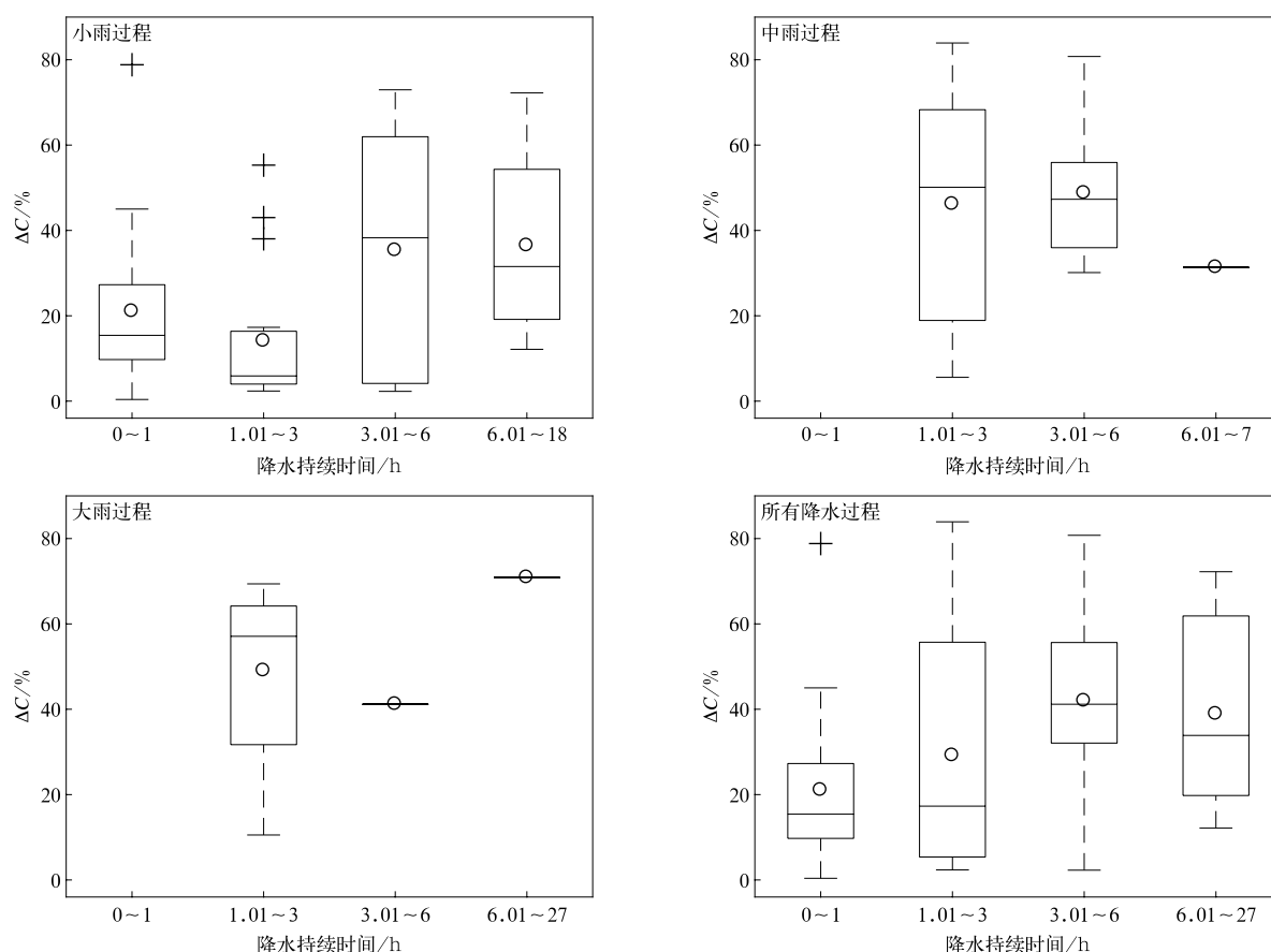
图 6 2014 年 3 月—2016 年 7 月北京降水后 \text{PM}_{2.5} 质量浓度减小个例中
