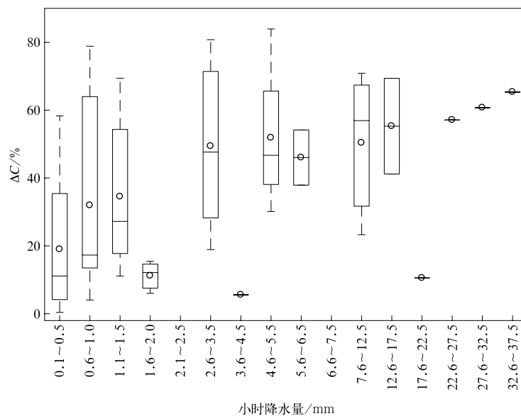
图 3 2014 年 3 月—2016 年 7 月北京降水后 PM 2.5 质量浓度减小 个例中不同小时降水量对应的 PM 2.5 清除率 (黑线代表中值,圆圈代表平均值,矩形框的上下边分别代表 上下四分位数,上下触须线分别代表最大值和最小值)
