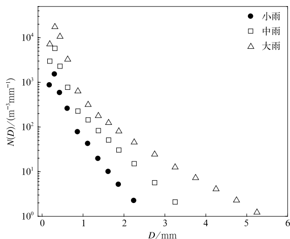
图4 北京小雨、中雨和大雨的平均雨滴谱分布
