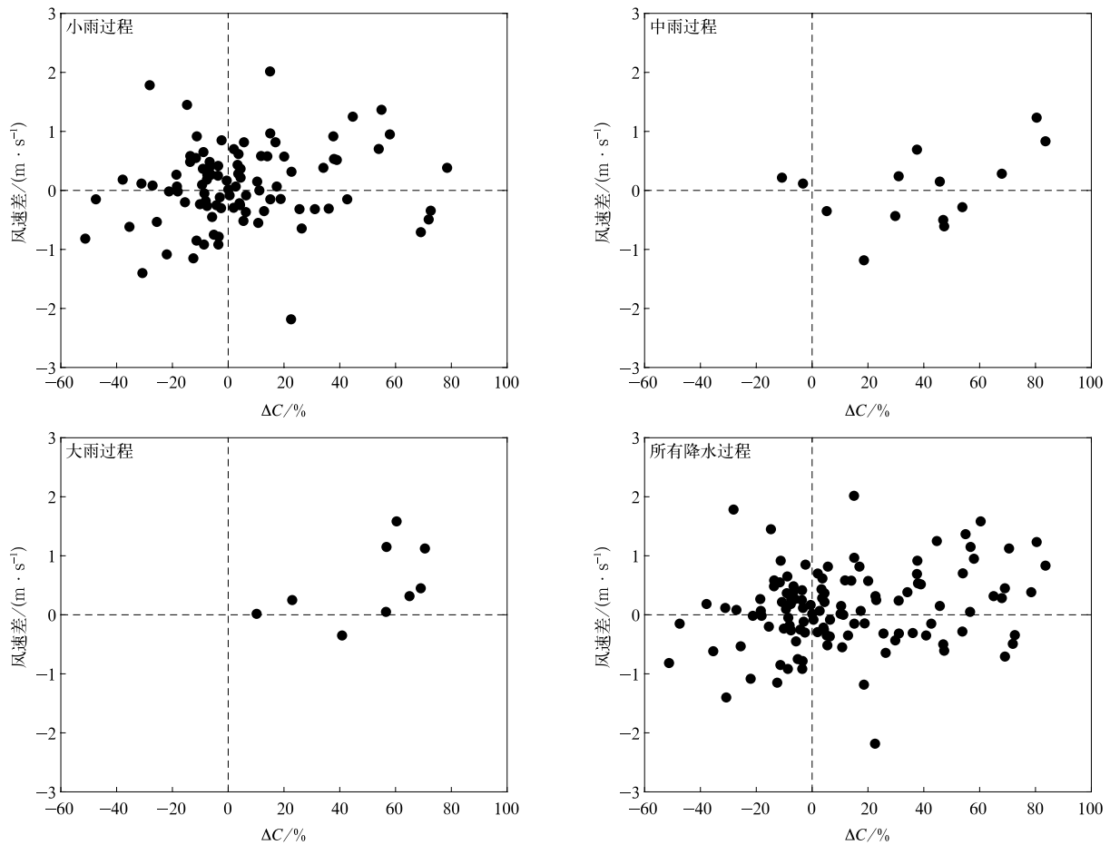
图8 2014年3月—2016年7月北京 \text{PM}_{2.5} 清除率和降水前后风速差的对应关系
