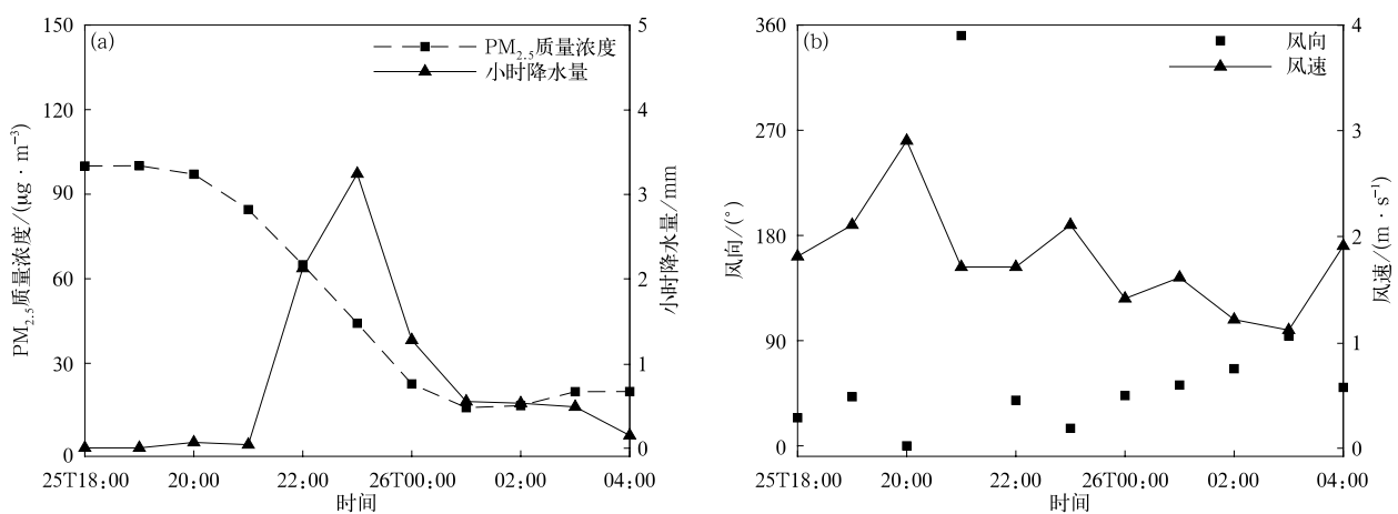
图9 2014年4月25—26日北京小雨过程 \text{PM}_{2.5} 质量浓度和
