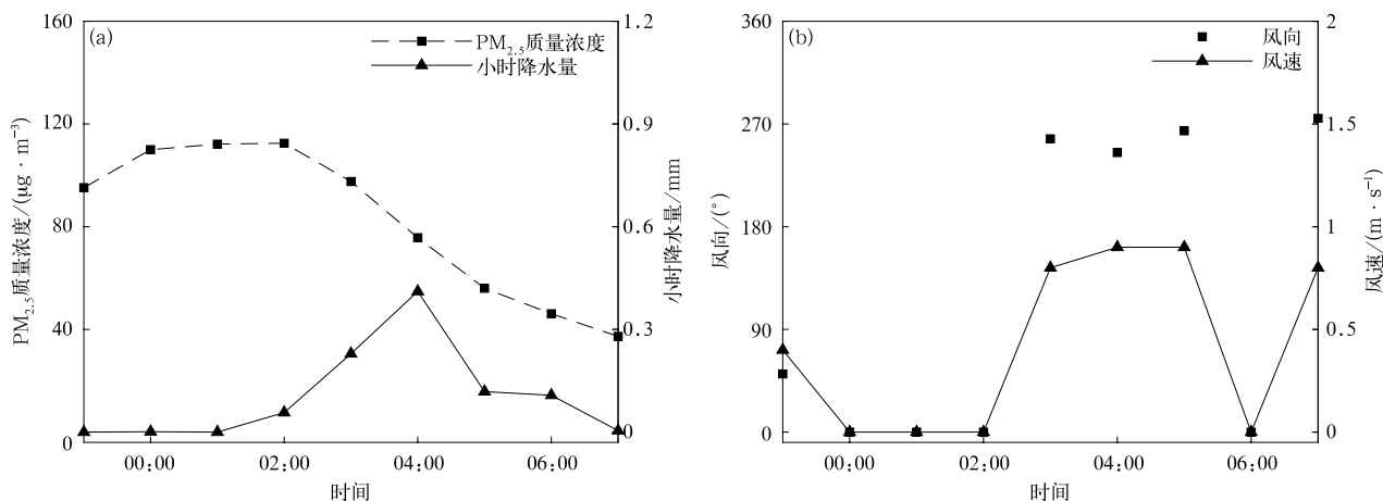
图10 2014年9月12日北京小雨过程 \text{PM}_{2.5} 质量浓度和小时降水量(a)以及风速和风向(b)随时间变化
