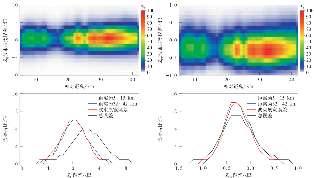
图 6 X-PAR 的 Z_H 和 Z_{DR} 波束展宽误差对比频次及误差量级占比
