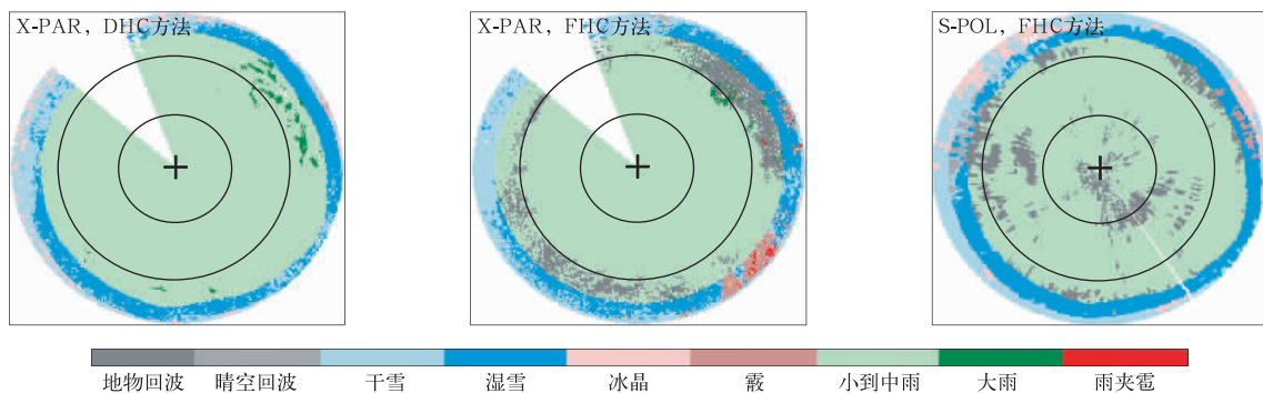
图 11 DHC 方法和 FHC 方法对于 2020 年 5 月 11 日 23:00 X-PAR 和 S-POL 探测水凝物相态识别结果
