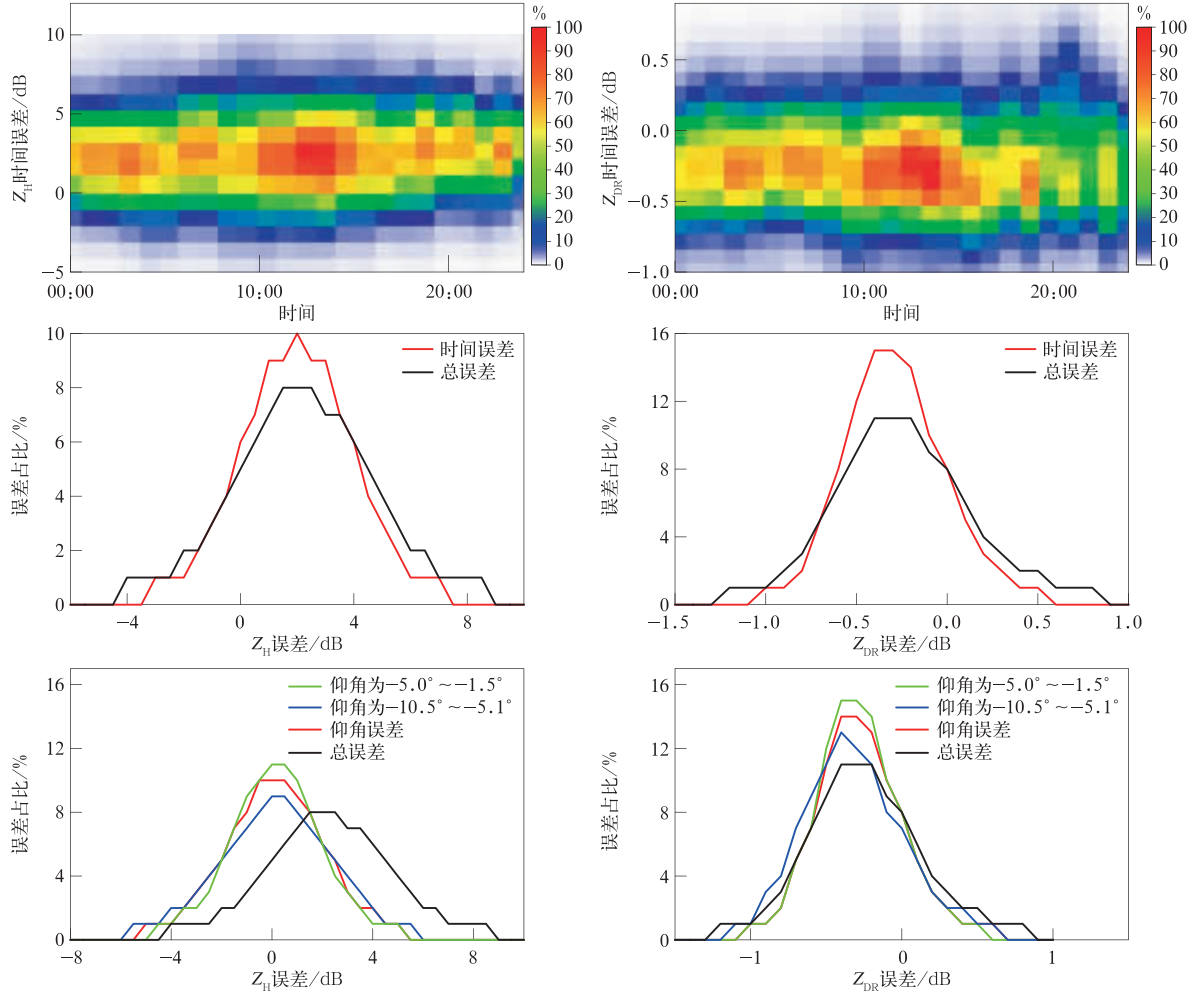
图4 X-PAR的 Z_H 和 Z_{DR} 标定误差对比频次及误差量级占比
