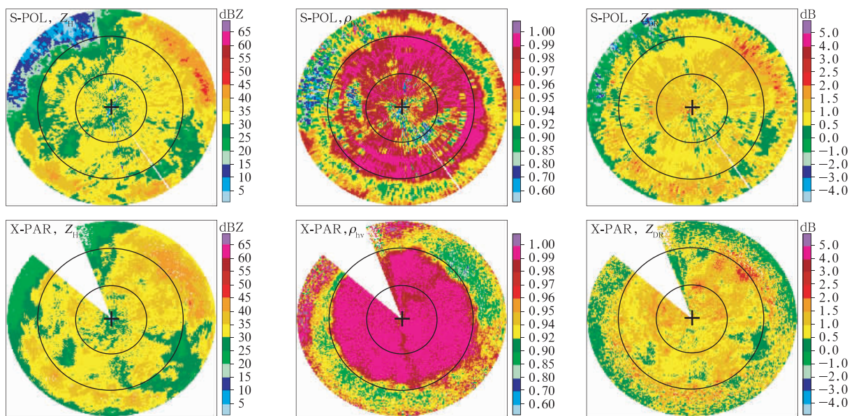
图 10 2020 年 5 月 11 日 23:00 X-PAR 和 S-POL 的 Z_H , \rho_{hv} 和 Z_{DR} 水平结构
