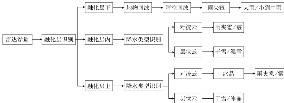
图 1 DHC 方法流程
