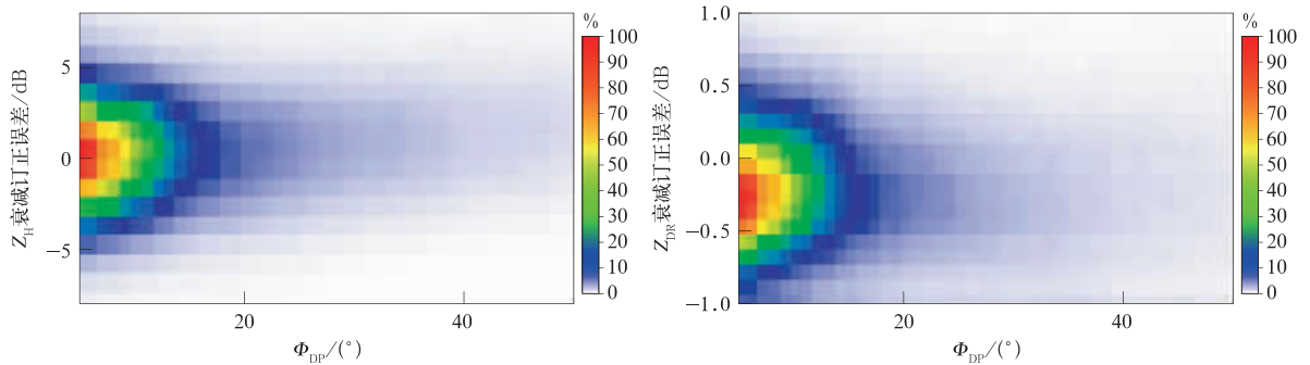
图5 X-PAR的 Z_H 和 Z_{DR} 衰减订正误差对比频次及误差量级占比
