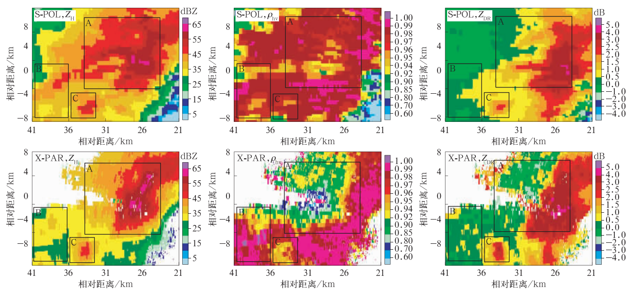
图 8 2020 年 3 月 18 日 09:37 X-PAR 和 S-POL 的 Z_H , \rho_{hv} 和 Z_{DR} 水平结构(6.3°仰角)
