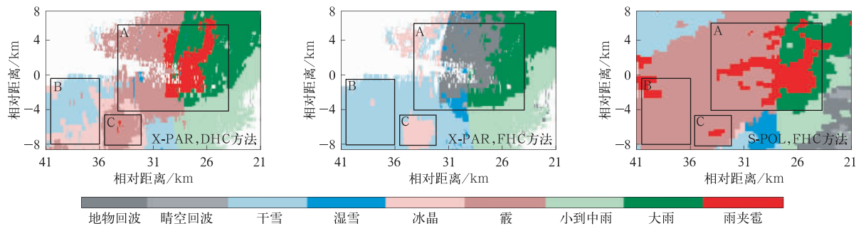
图 9 DHC 方法和 FHC 方法对于 2020 年 3 月 18 日 09:37 X-PAR 和 S-POL 探测水凝物相态识别结果(6.3°仰角)
