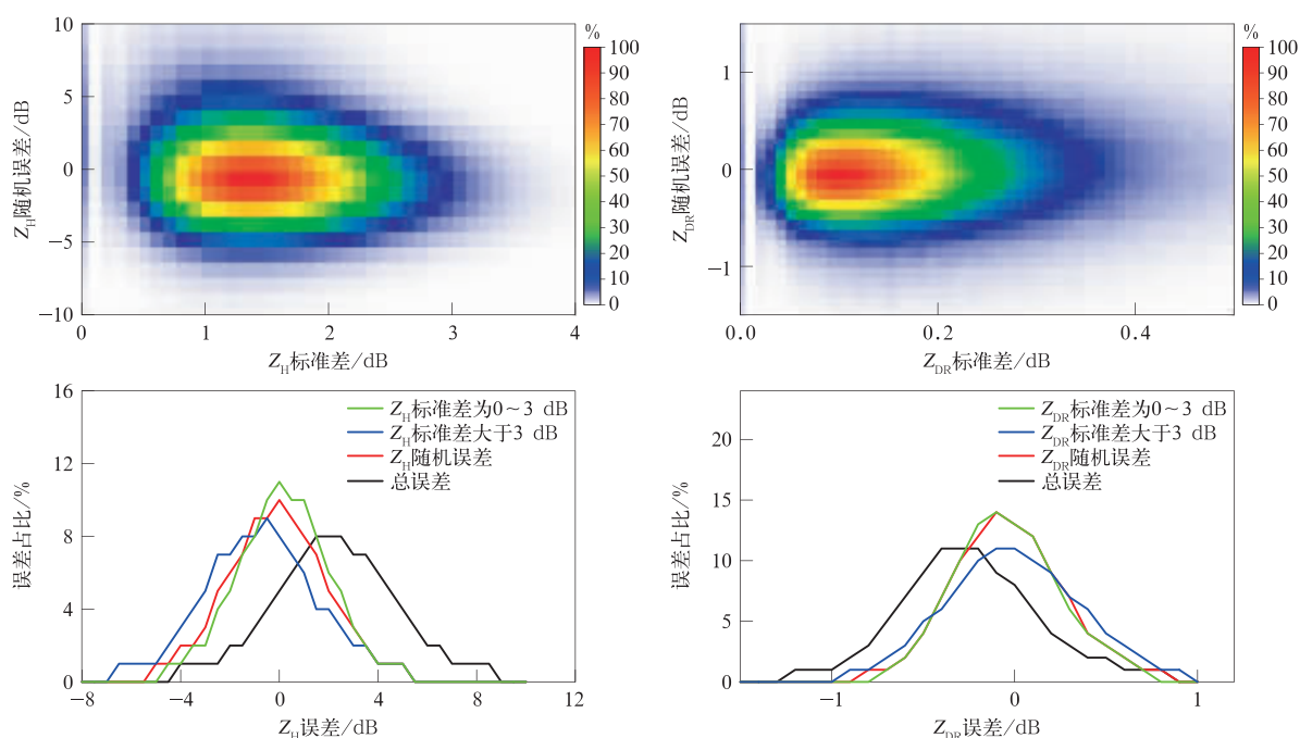
图 3 X-PAR 的 Z_H 和 Z_{DR} 随机误差对比频次及误差量级占比
