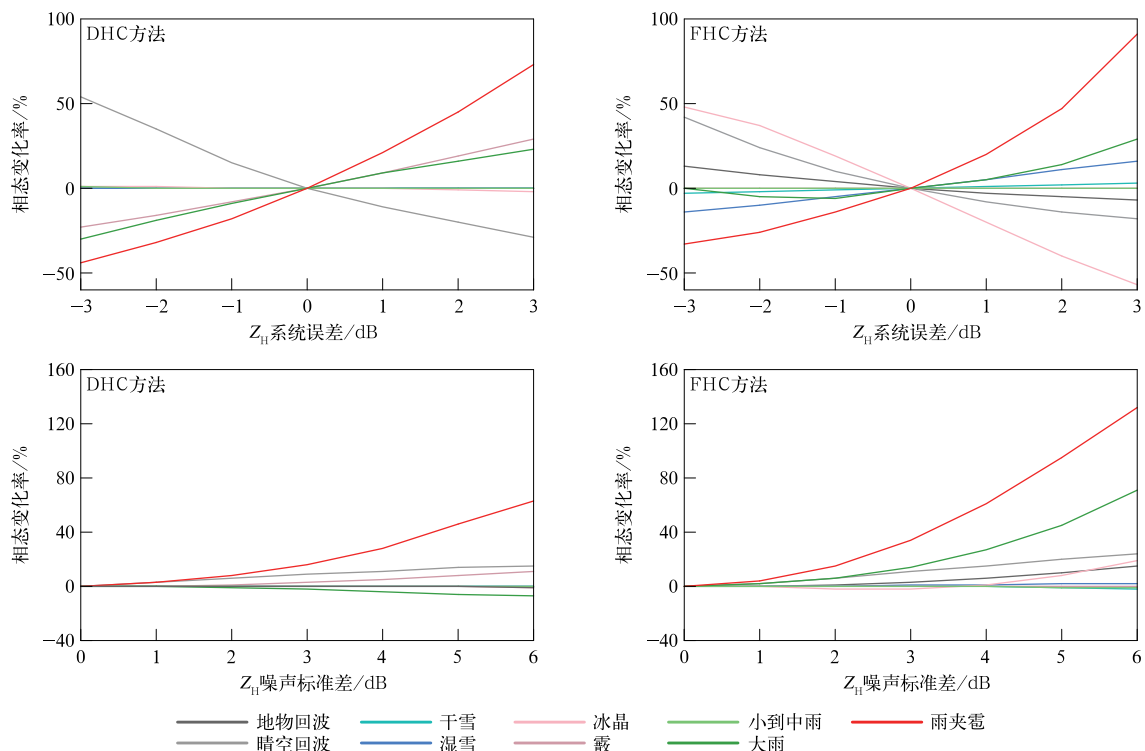
图7 向 Z_H 分别引入系统误差和随机误差后相态变化率
