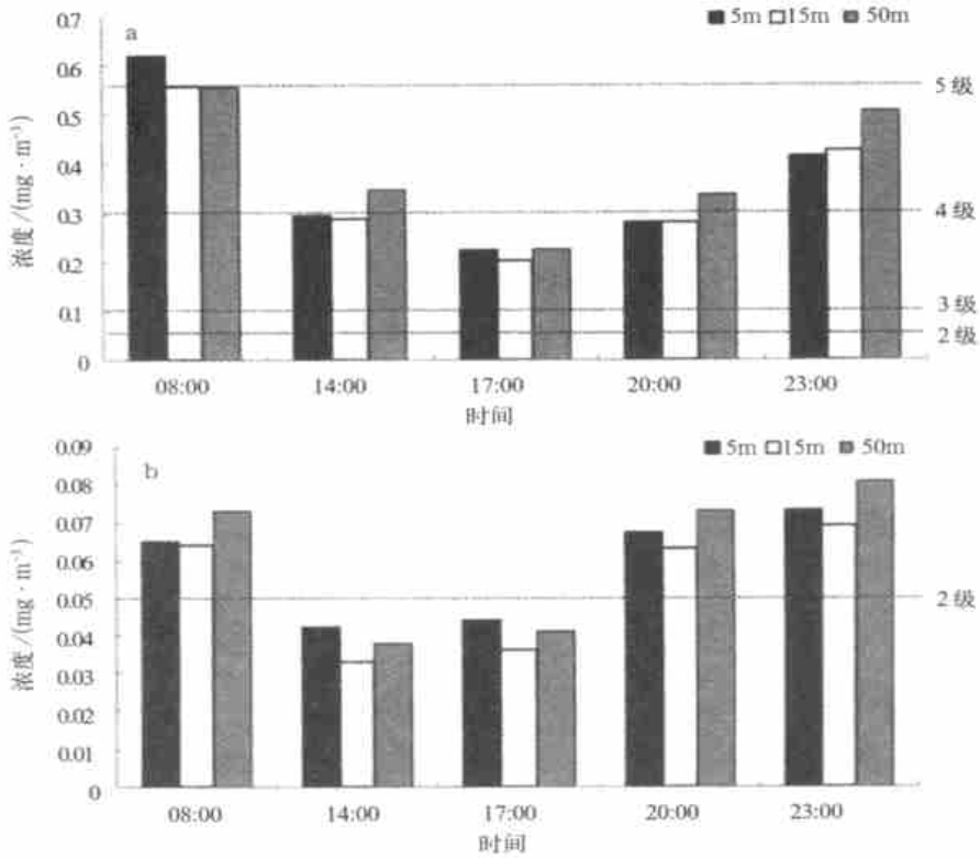
图 4 静稳天气(a)与利于扩散天气(b)条件下不同高度处 \text{NO}_x 浓度对比
