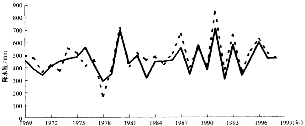
图1 DAMSM 模式对 1969 ~ 1998 年降水量的拟合预报与实际降水量的比较 (实线表示 DAMSM 模式降水量,虚线表示实际降水量)
