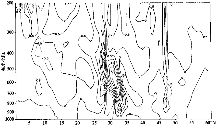
图2 7月22日00:00 UTC沿114°E的垂直速度剖面图(单位: 10^{-1} m/s)
