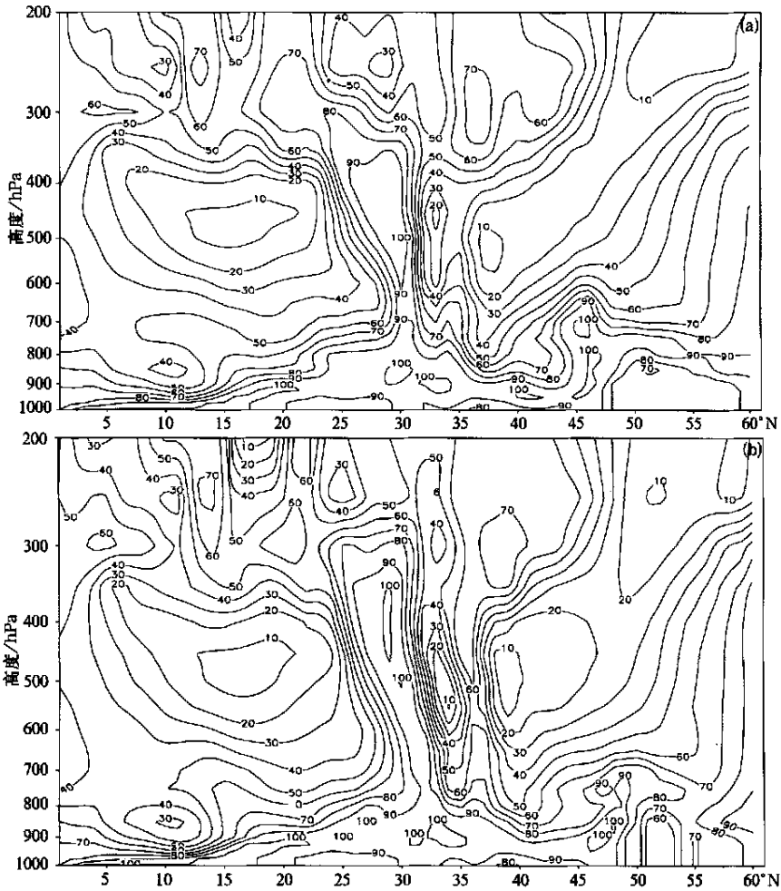
图 1 1998 年 7 月 22 日 00:00 UTC 相对湿度沿 114°E 的剖面图 (a) 方案 1, (b) 方案 2
