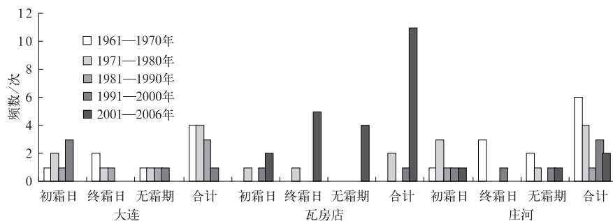
图 1 大连地区各站不同年代异常霜冻事件出现的频数
