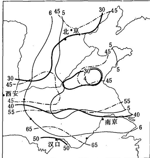
图2 7—8月平均距平百分率(粗实线), 平均年际变化百分率(点划线)和日降水量≥10mm 平均间隔日数的平均距平(细实线)
