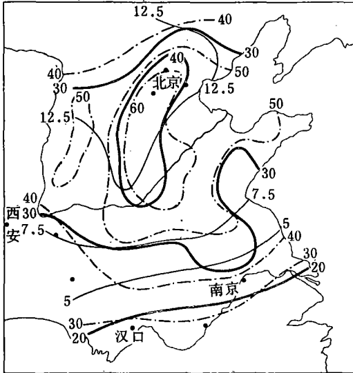
图1 3—6月平均距平百分率(粗实线), 平均年际变化百分率(点划线)和日降水量≥5mm 平均间隔日数的平均距平(细实线)
