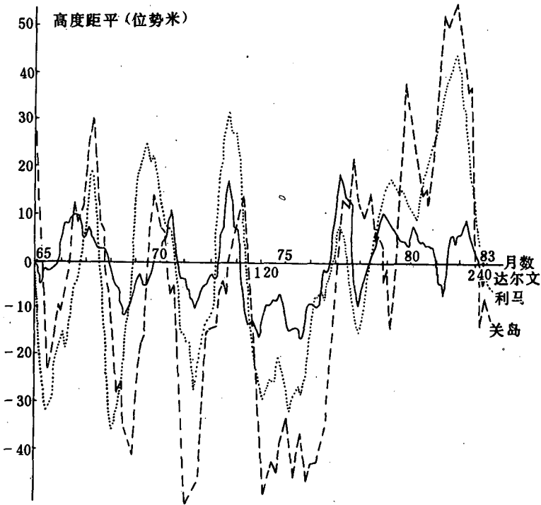
图1 1964—1984年三站12个月滑动的月平均高度距平曲线。
