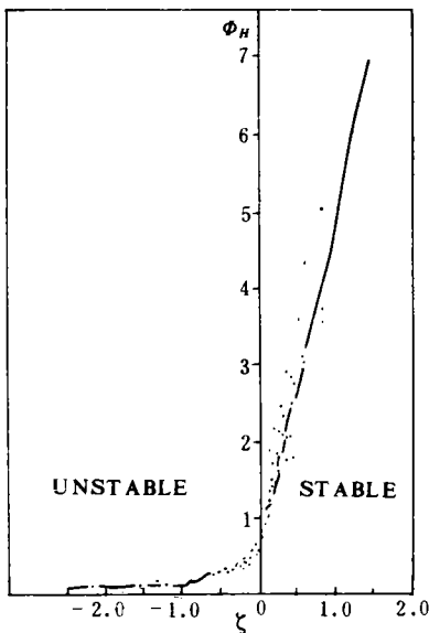
图 2 \Phi_H(\zeta) 与 \zeta 关系图 (实点为 Businger 等人的资料)
