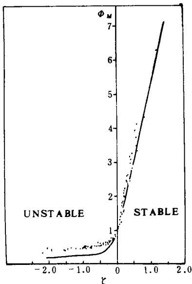
图 1 \Phi_M(\zeta) 与 \zeta 关系图 (实点为 Businger [3] 等人的资料)
