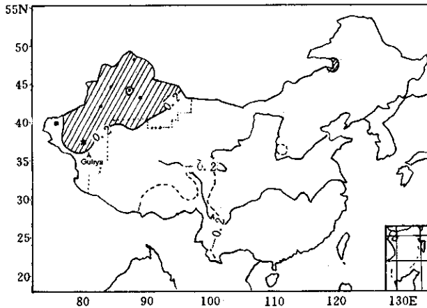
图3 古里雅冰芯 \delta^{18}\text{O} 与气温的相关系数
