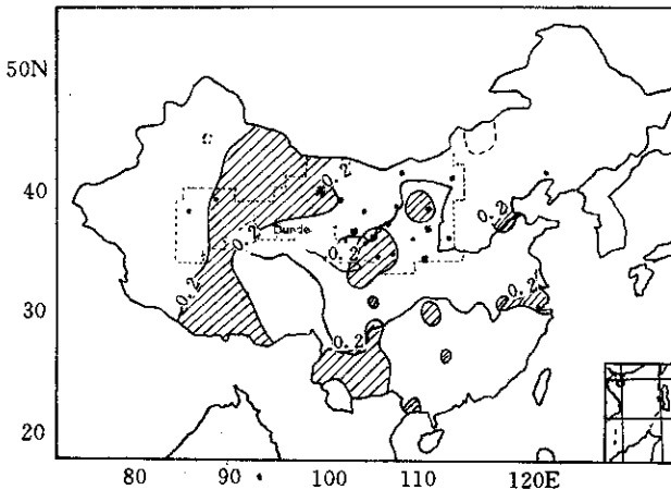
图2 敦德冰芯 \delta^{18}\text{O} 与气温的相关系数
