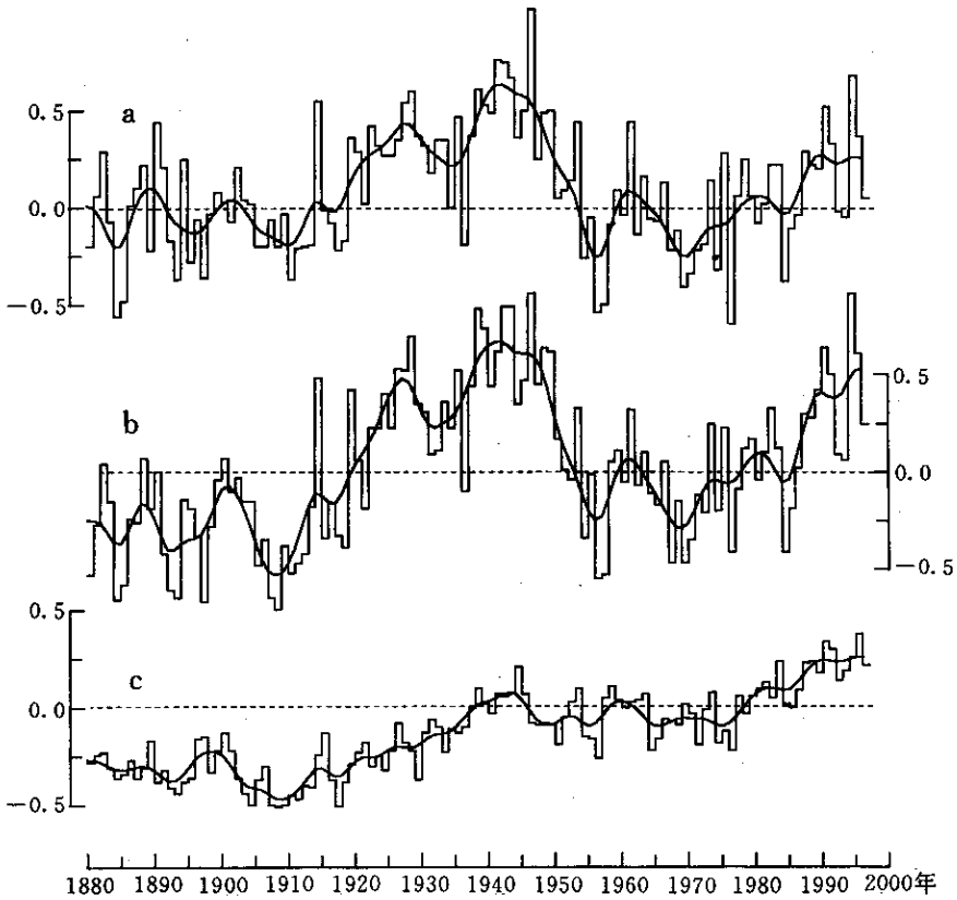
图5 (a)1990年给出的年平均中国气温距平 [1] (b)本文的年平均中国气温距平序列(c)全球年平均气温距平序列(纵坐标表示,单位:°C)
