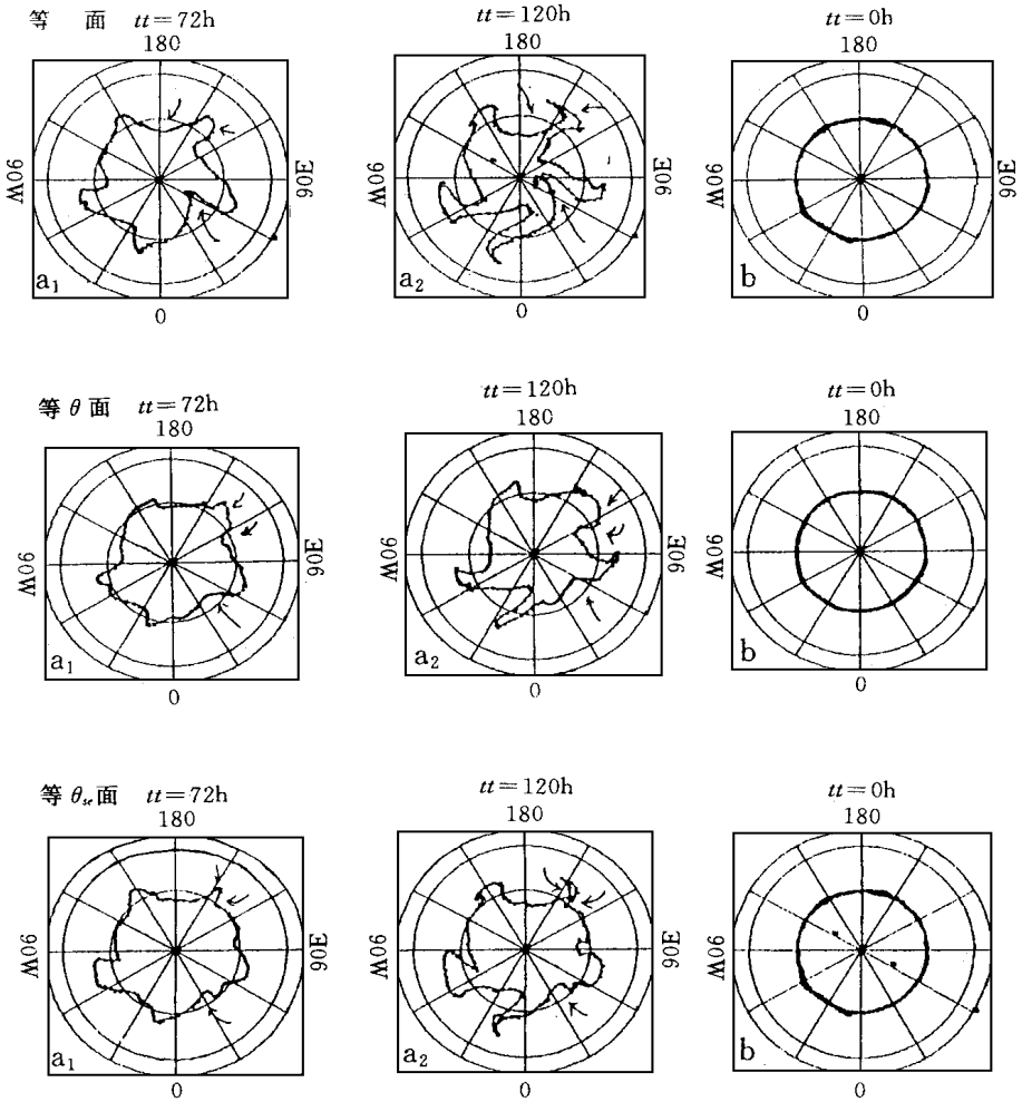
图1 1991年7月1~5日以60°N纬圈为初始物质线的轨迹积分 ( tt 为积分时间, a. dc=7 格距 b. dc 取足够大)
