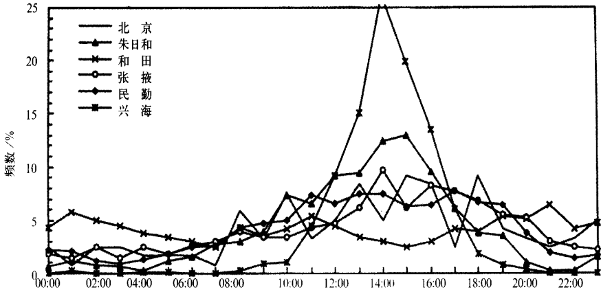
图 2 北京等 6 个代表站 1 h 间隔的沙尘暴频数分布
