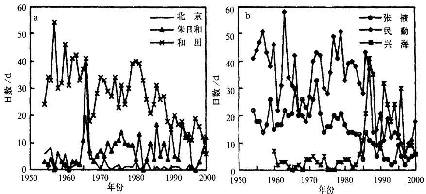
图 4 北京等 6 个代表站 1954 ~ 2000 年沙尘暴日数的年际变化
