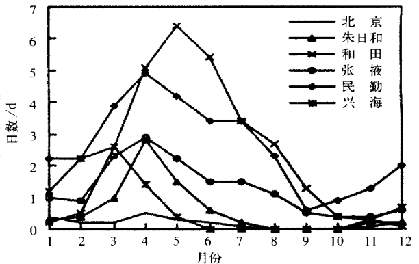
图 3 北京等 6 个代表站沙尘暴日数的季节变化 例如北京主要集中在春季(3 ~ 5 月),期间沙尘暴日数占全年总出现日数的 52.6%;朱日和与北京类似;青海兴海主要集中在冬末春初(2 ~ 4 月),期间沙尘暴日数占全年总出现日数的 70.0%;和田、民勤和张掖等地春夏季(3 ~ 8 月)沙尘暴都很频繁。
