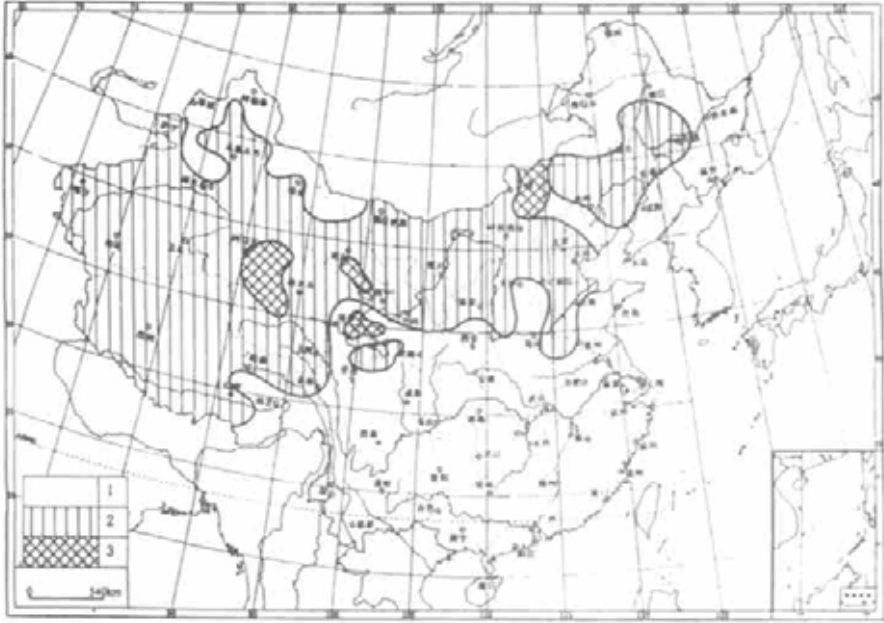
图 5 1954~2000 年沙尘暴日数变化趋势的全国分布(1.不变,2.减少,3.增加)
