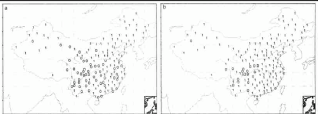
图 4 我国年平均气温线性趋势分布图(图中标“1”为上升趋势,“0”为下降趋势) (a) 1951 ~ 1990 年, (b)1951 ~ 2000 年
