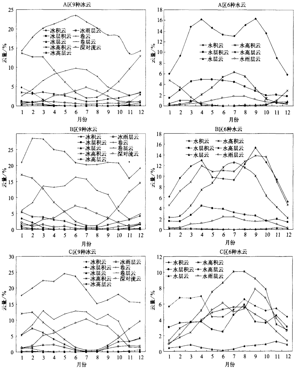
图4 1984年1月~1998年12月A,B,C各区9种冰云和6种水云云量季节变化
